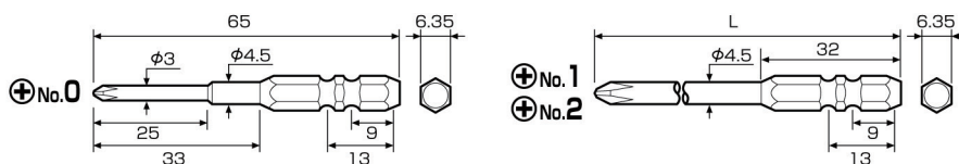
■ ハイパービット 2本組・5本組（段付・W溝タイプ）
