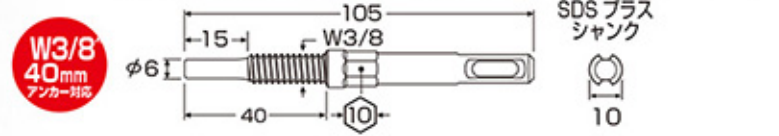
AEB-340SDS アンカー抜きビット SDSプラスシャンク
