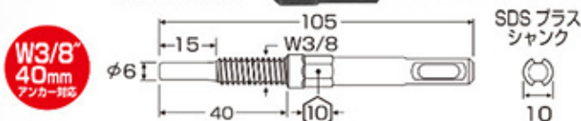
■ AEB-340SDS アンカー抜きビット SDSプラスシャック
