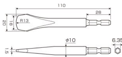
AHC-1511 コインドライバービット
