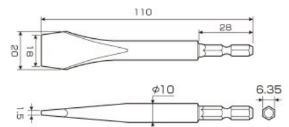
AHF-1511 水栓ドライバービット
