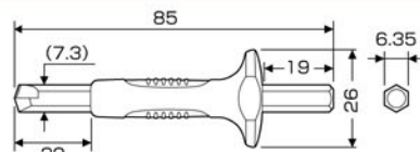
AK-22N ネジとりビット
