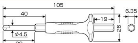
AK-22NS ネジとりビット スリムタイプ
