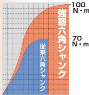
六角シャンクねじり強度比較表 (当社比)
